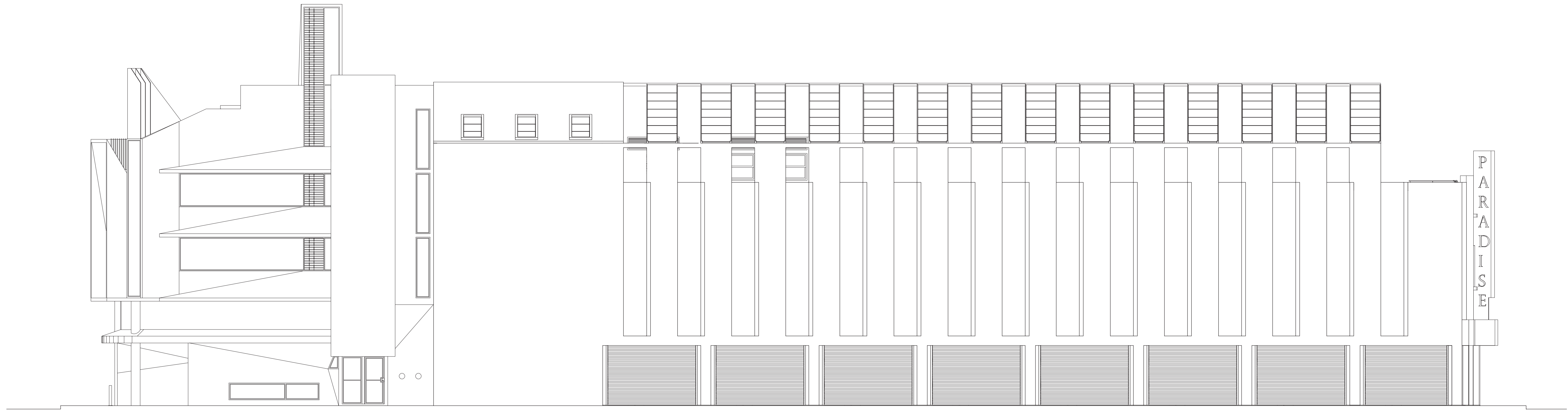
1' 6' 16' 24' ESCALA: 1/8" = 1' FACHADA SUR
