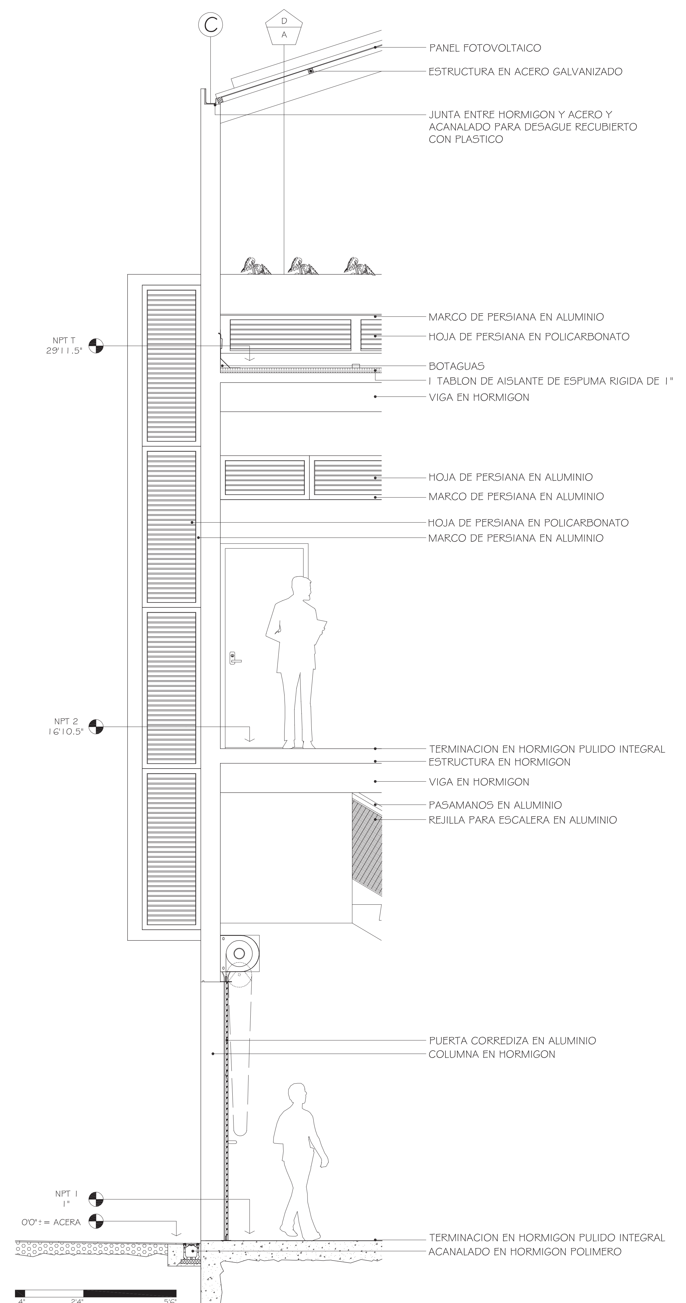
ESCALA: 1/2" = 1' FACHADA EN SECCION
