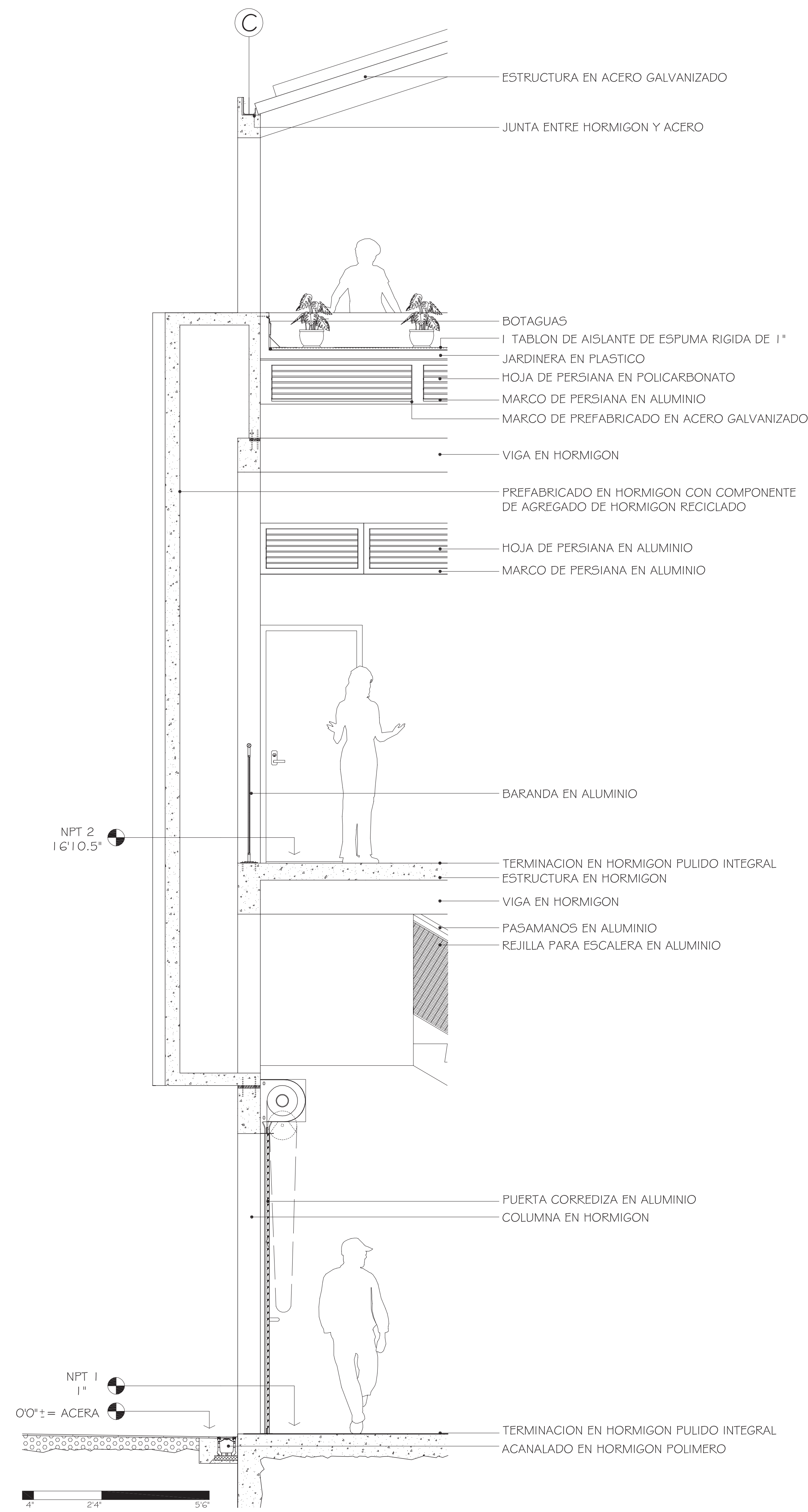
ESCALA: 1/2" = 1' SECCION DE PARED
